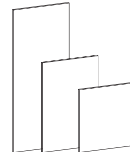
Задняя стенка ЛДСП NLN 363 853 76x1,8xh193 NLN 363 852 76x1,8xh116 NLN 363 851 76x1,8xh77
