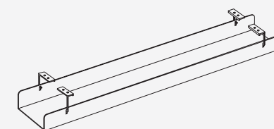
Лоток широкий на 2 стола CBM 336 111 80x16xh5,5 CBM 336 112 100x16xh5,5 CBM 336 113 120x16xh5,5 CBM 336 114 140x16xh5,5 CBM 336 115 160x16xh5,5
